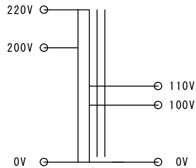
結線図
