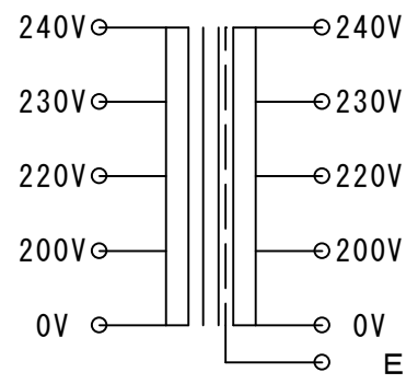
結線図
