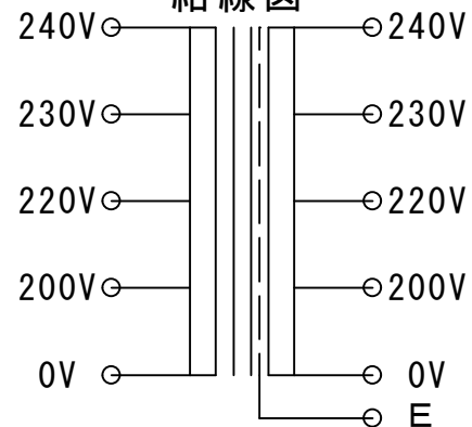
結線図
