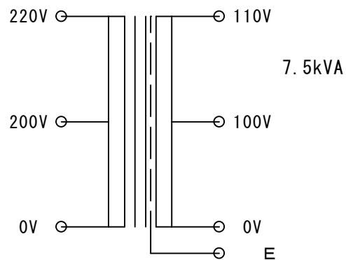
結線図
