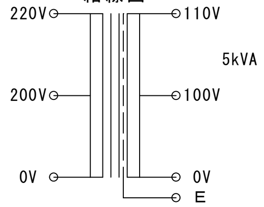
結線図
