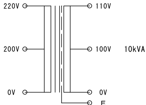
結線図
