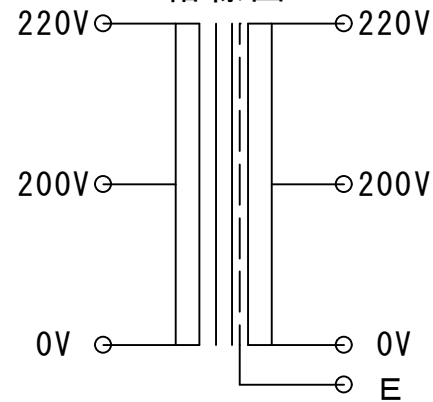
結線図
