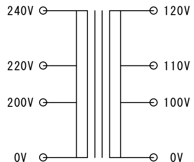
結線図
