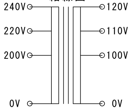
結線図
