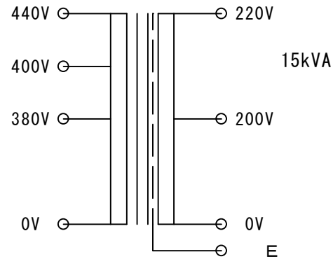
結線図
