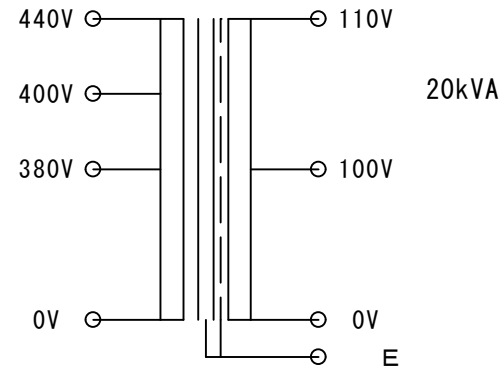
結線図
